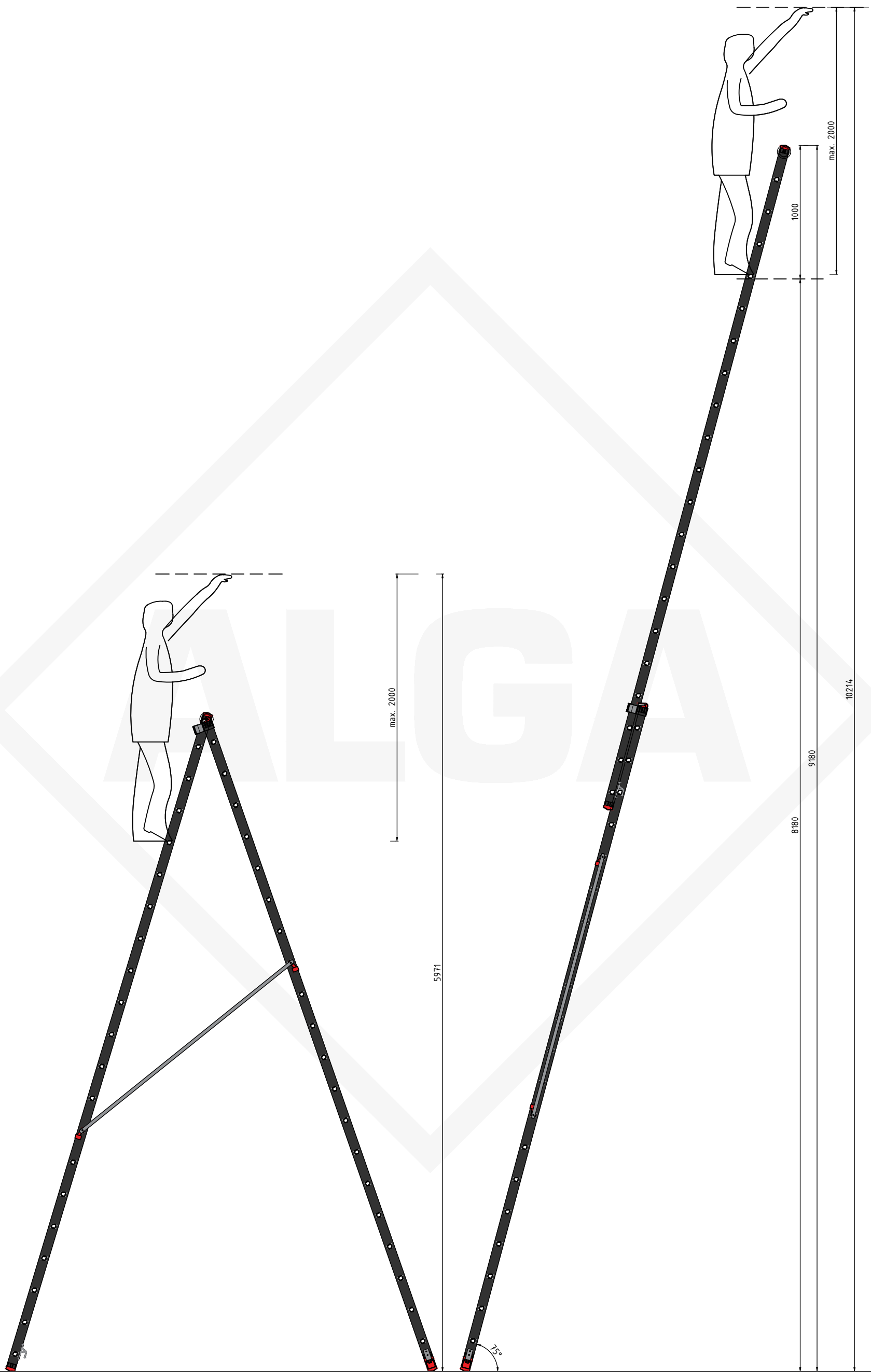
Type. MRL220 Artikel nr. 100220
