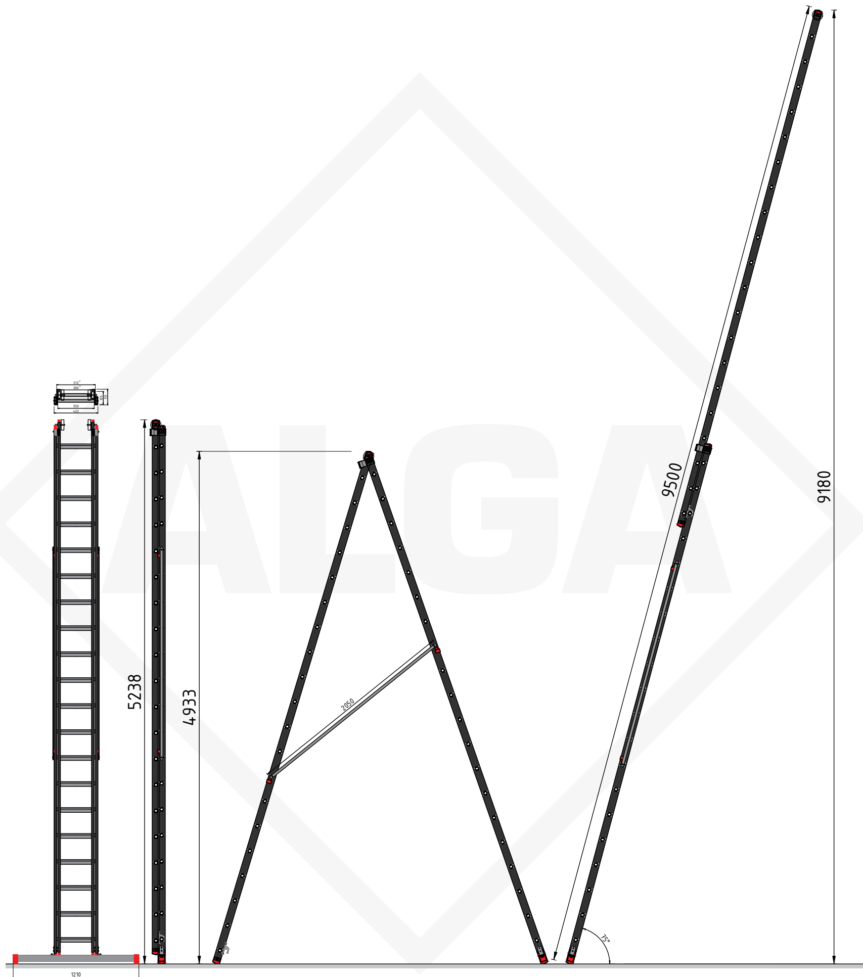
Type. MRL220 Artikel nr. 100220
