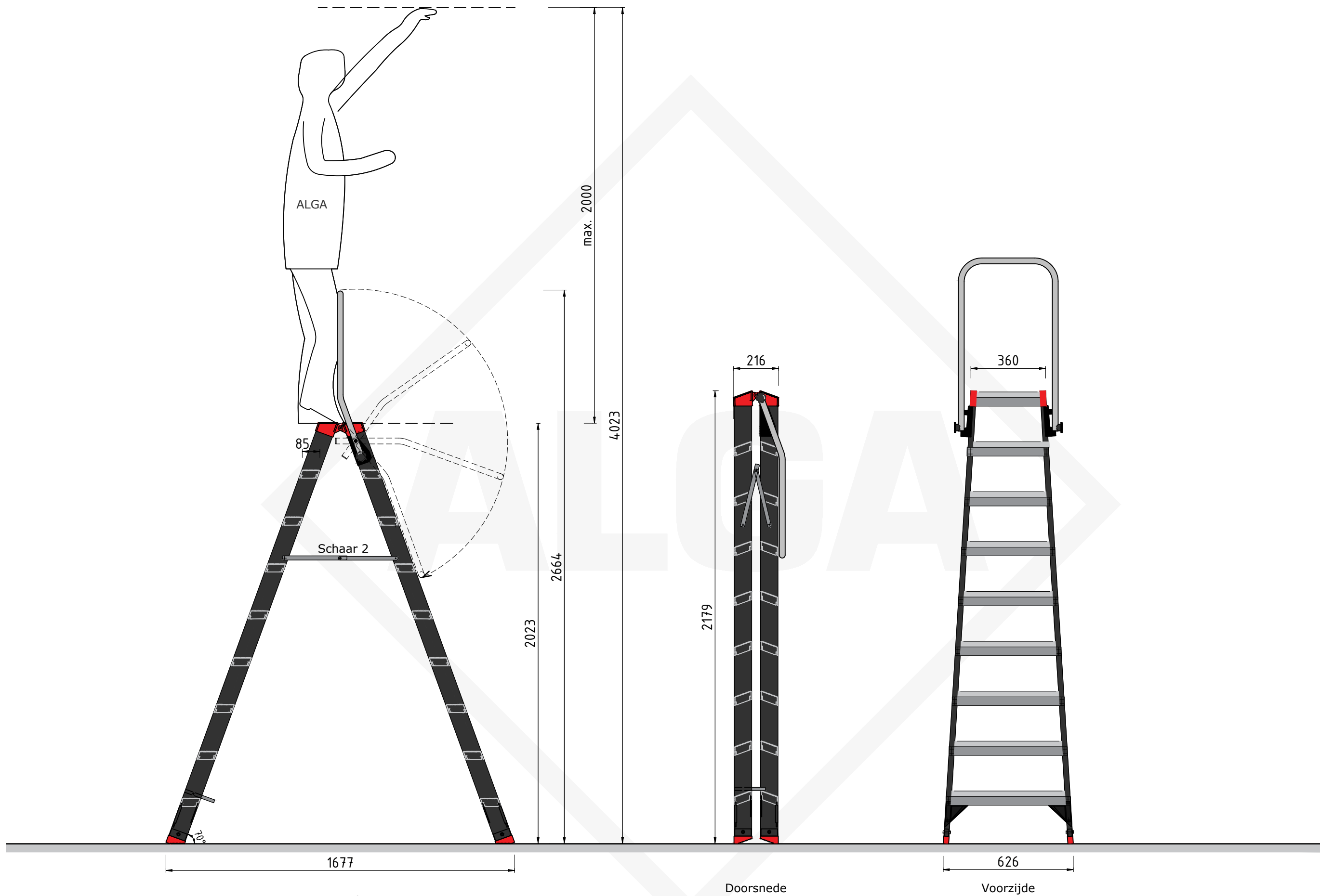
Doorsnede
