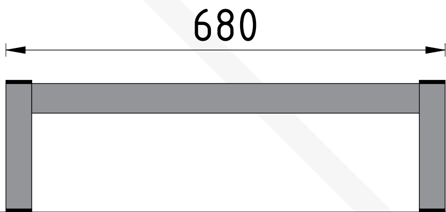
vooraanzicht
