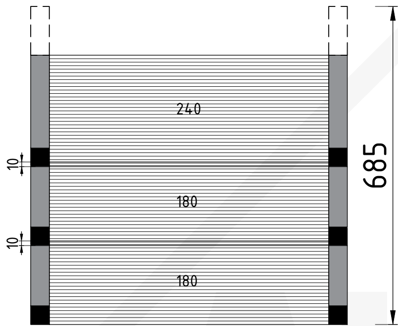
bovenaanzicht
