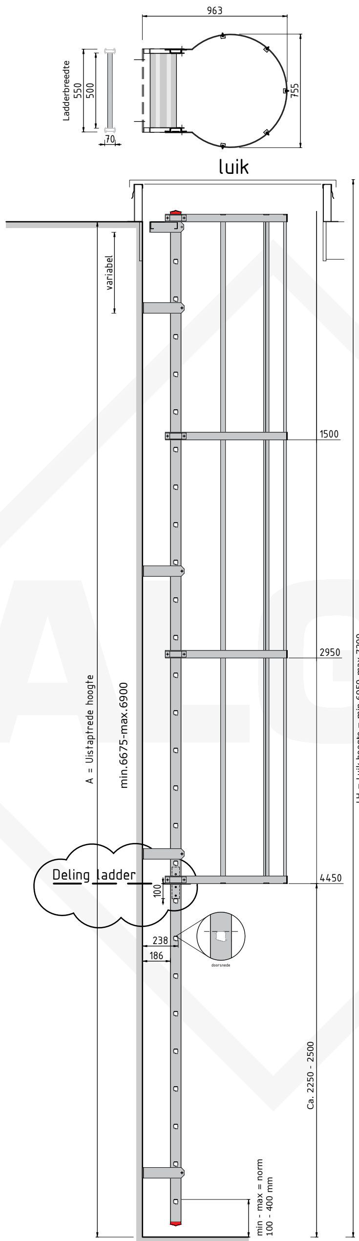
Doorsnede
